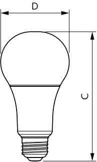
A21 120V 18.5-150W 2150lm 2700K E26 ND
