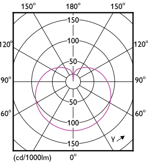
LEDbulb A21 E26 2150lm FR
