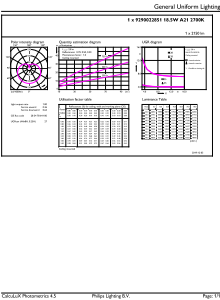
LEDbulb 18,5W A21 E26 927 FR
