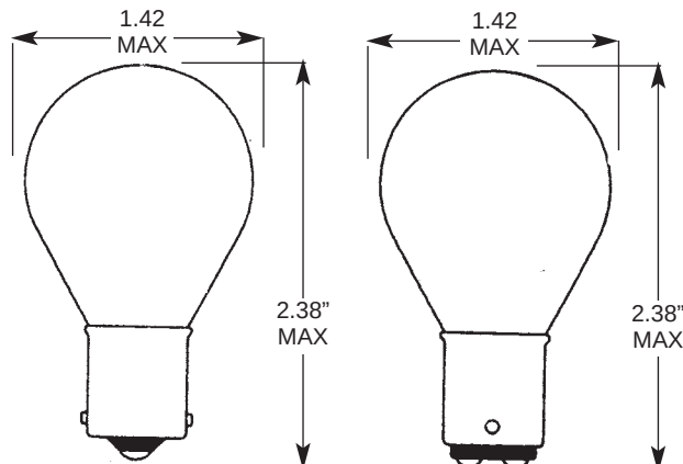
S. C. BAYONET BASE
