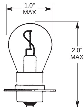
S. C. PREFOCUS BASE
