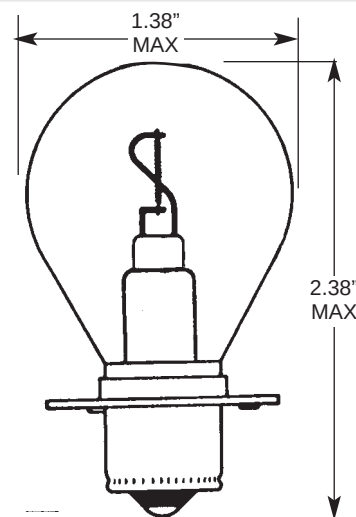
S. C. PREFOCUS BASE
