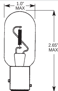
D.C. INDEXING BASE
