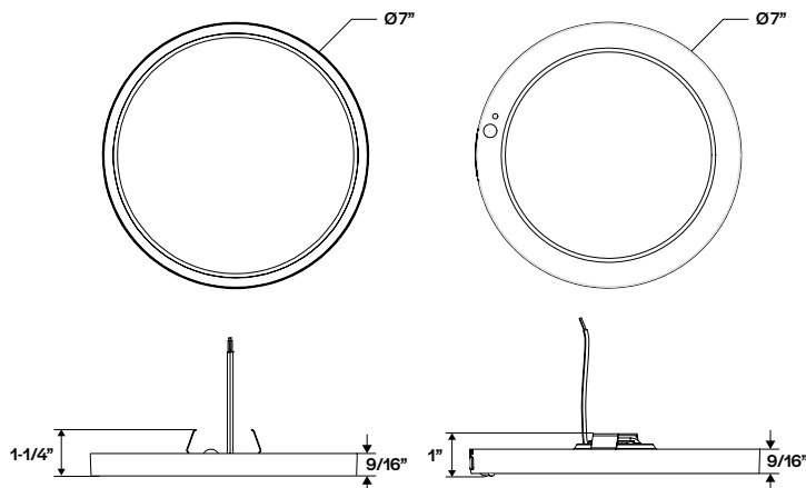
DSK-7-CS-120V
