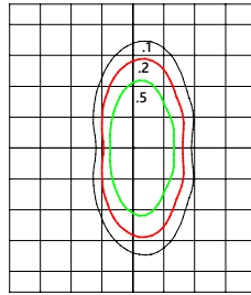
ERL1 Type II Narrow Visual Comfort Lens 14601 Lumens 4000K ERL1_16J740___IES
