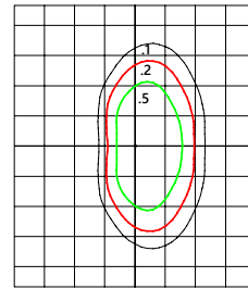
ERL1 Type II Visual Comfort Lens 14601 Lumens 4000K ERL1_16K740___IES
