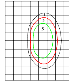
ERL1 Type III Visual Comfort Lens 14601 Lumens 4000K ERL1_16L740___IES
