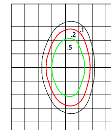
ERL1 Type II-EB Visual Comfort Lens 14601 Lumens 4000K ERL1_16N740___IES
