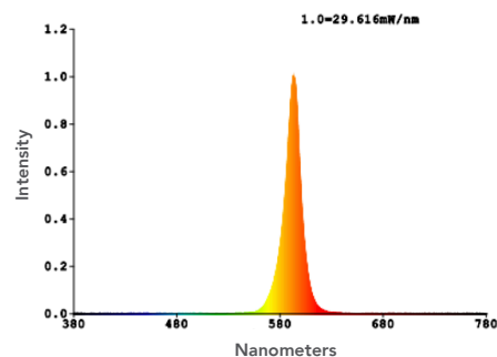
Amber (-AMB) Spectral Output
