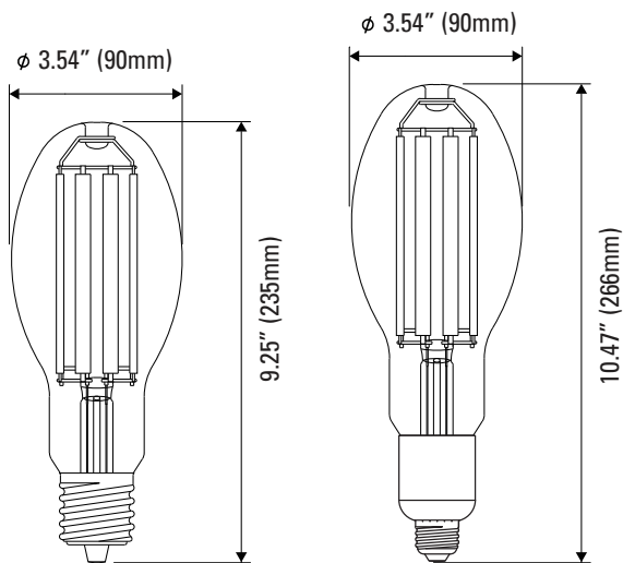
ED28 Lamp 25 Watt: 0.37-lb 30 Watt: 0.44-lb 40 Watt: 0.46-lb
