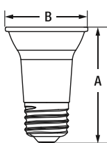
PAR16 E26
