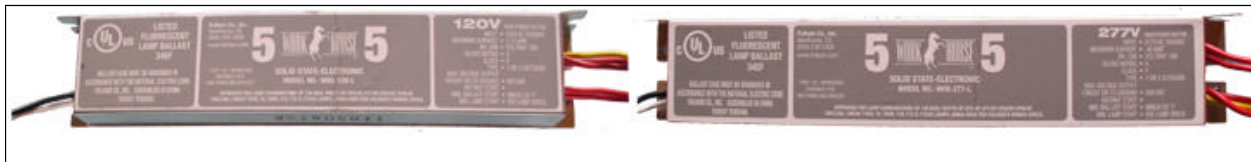
WH5-120-L (1.7" x 1.0" x 8.5")
