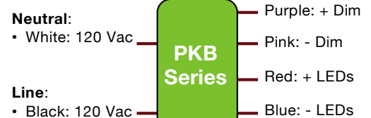
Wiring Diagrams
