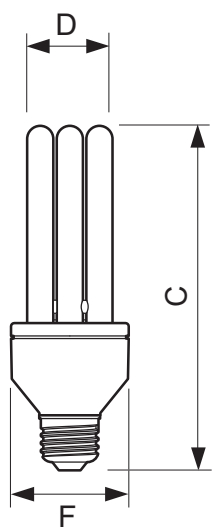
Universals 14W Med SLS ALTO 1CT
