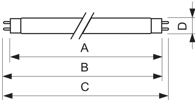
TL-D 18W/865 1SL
