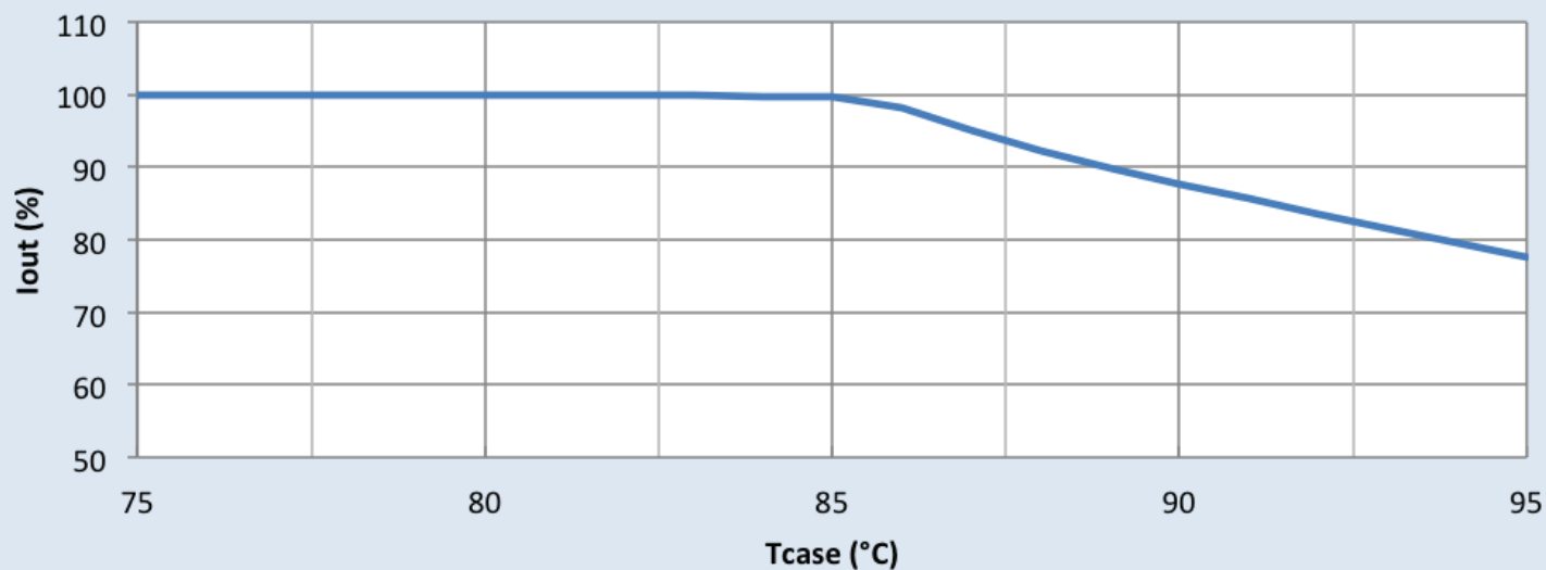
Iout (%) vs. Tcase
